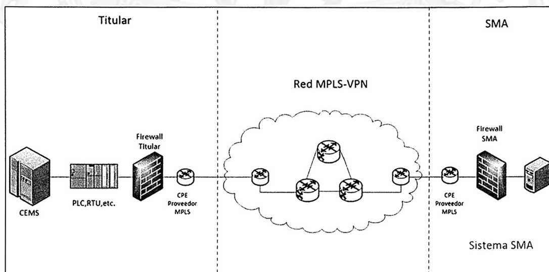
Figura 2: Diagrama de conexión con PLC Espejo
