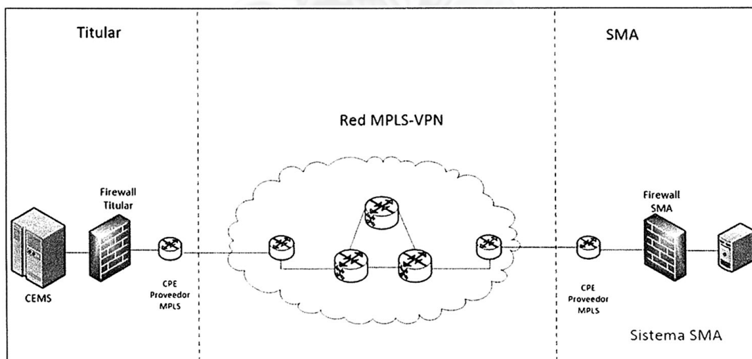
Figura 1: Diagrama de conexión Directa
