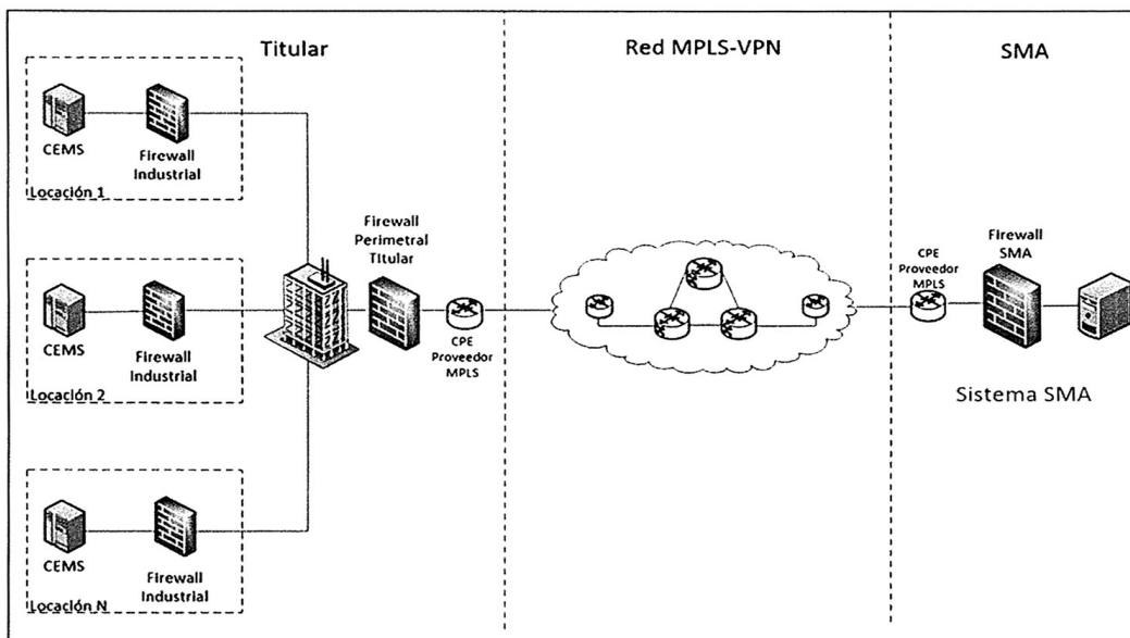
Figura 3: Diagrama de conexión concentrada (varias locaciones de un mismo titular)
